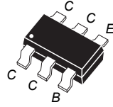
SOT-26 CASE
