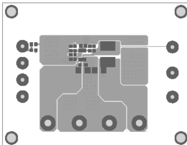
Figure 2—Top Layer
