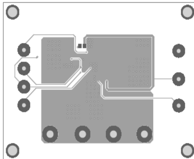
Figure 4—Bottom Layer
