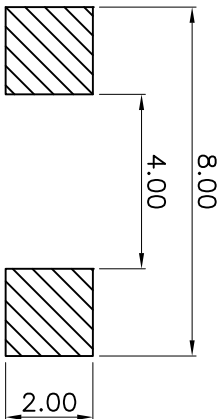
PCB Layout(Pattern side)
