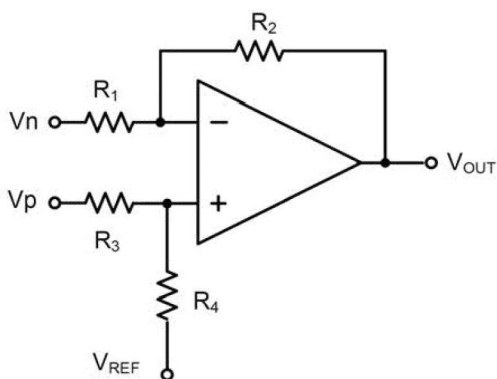
图 4, 差分放大器
