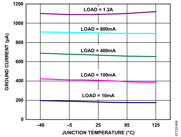
图8. 接地电流与结温的关系
