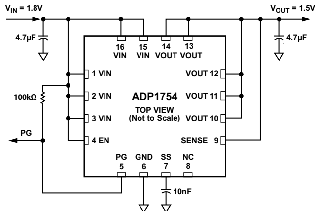
图1. 提供1.5 V固定输出电压的ADP1754
