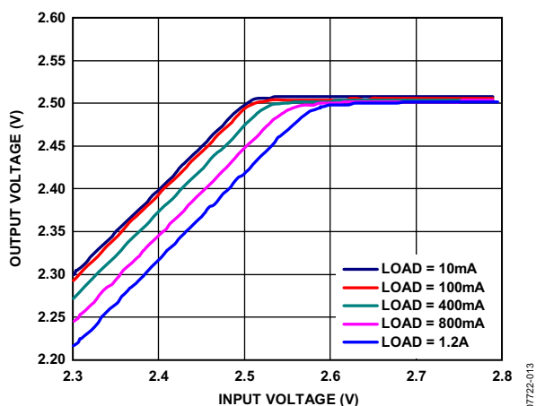
图13. 低压差下输出电压与输入电压的关系( V_{\text{OUT}} = 2.5 \text{ V} )
