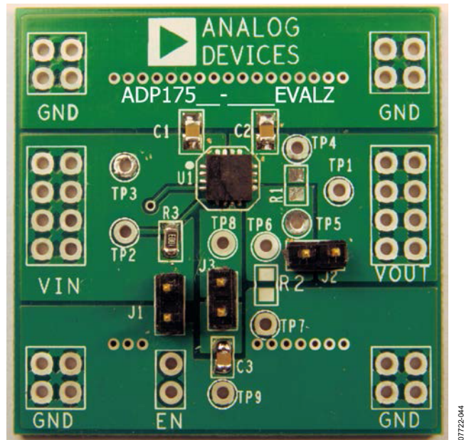
图46. 评估板
