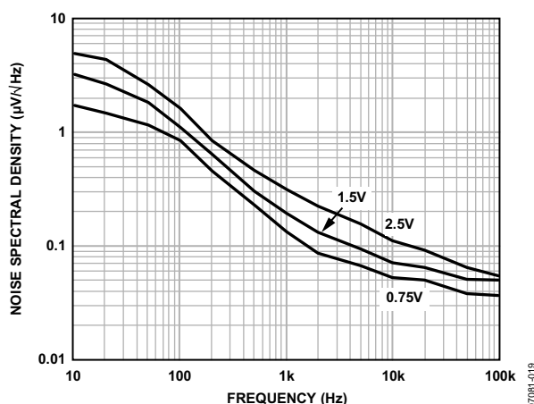
图19. 噪声谱密度与输出电压的关系 ( I_{LOAD} = 10 \text{ mA} )
