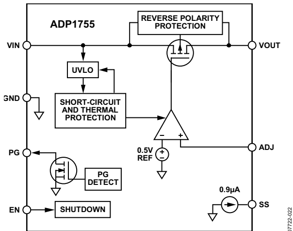
图25. ADP1755内部框图
