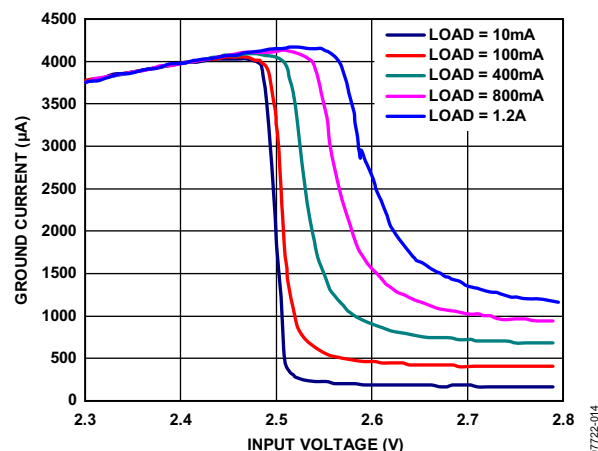
图14. 低压差下接地电流与输入电压的关系( V_{\text{OUT}} = 2.5 \text{ V} )
