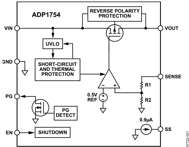
图24. ADP1754内部框图
