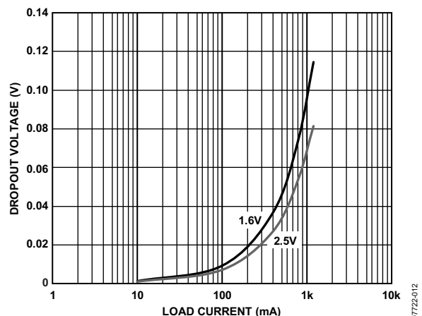
图12. 压差与负载电流的关系( V_{\text{OUT}} = 1.6 \text{ V} , 2.5 \text{ V} )
