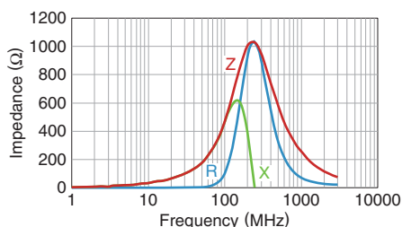
MMZ1608Q471BTA00
