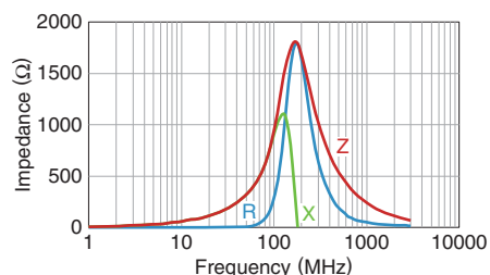
MMZ1608Q102BTA00
