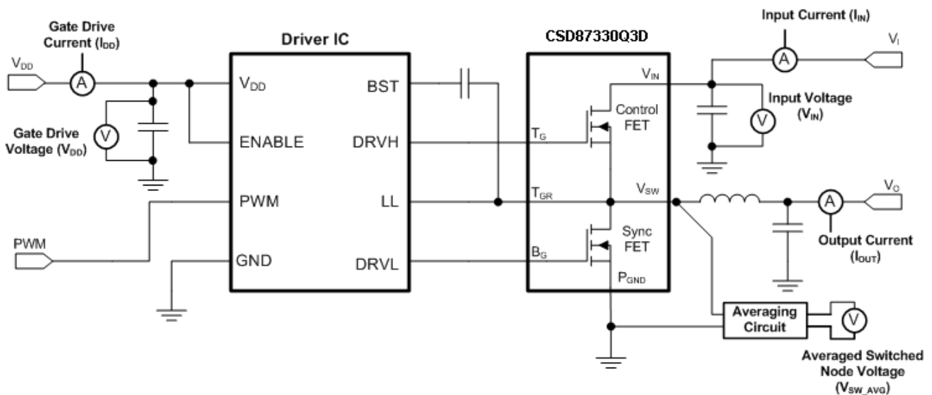
Figure 32. 典型应用
