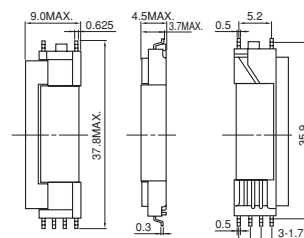
DIMENSIONS (mm) 外形寸法図
