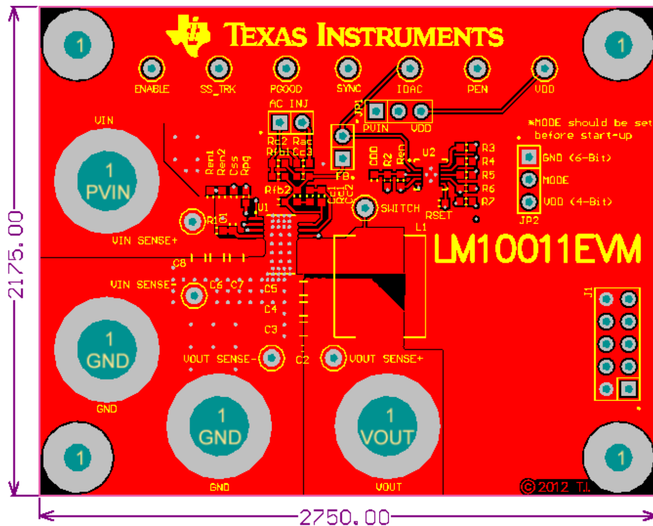
图 14. Typical Top Layer Layout
