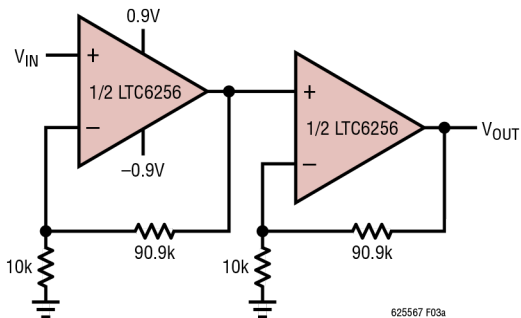
200kHz 130 \mu A 100 倍增益放大器
