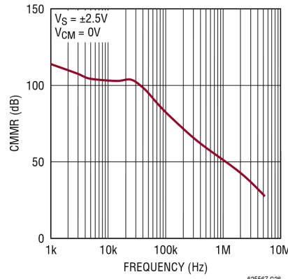
共模抑制比与频率的关系
