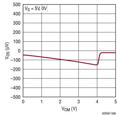
V_{OS} 与共模电压的关系
