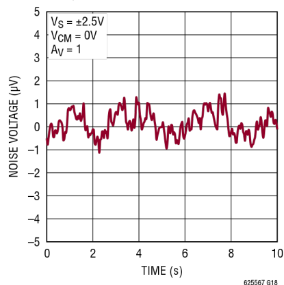
0.1Hz 至 10Hz 输出电压噪声
