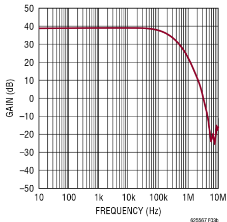
图 3.100 倍增益放大器 (3dB 带宽为 200kHz, 130 \mu A 电源电流)
