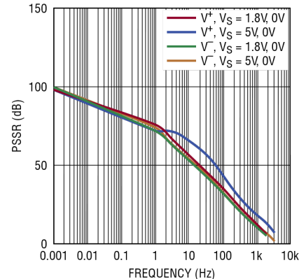
电源抑制比与频率的关系
