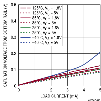
输出饱和电压与负载电流的关系 (输出低电平)
