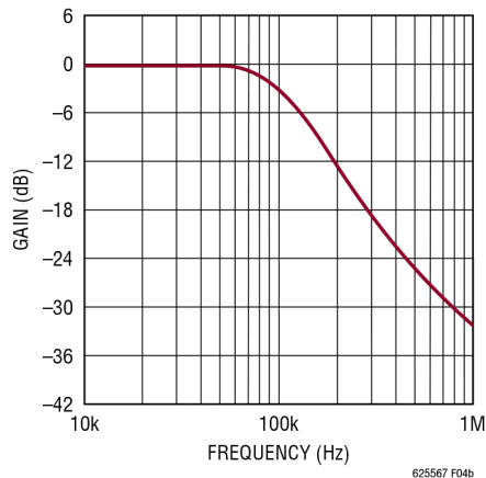
频率响应
