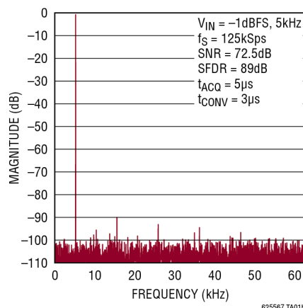
LTC6255 驱动 LTC2361 ADC
