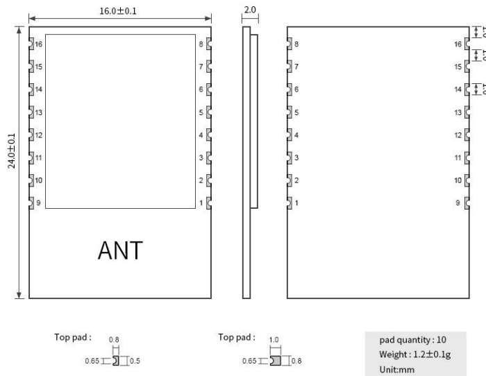
图 3-1 机械尺寸与引脚定义
