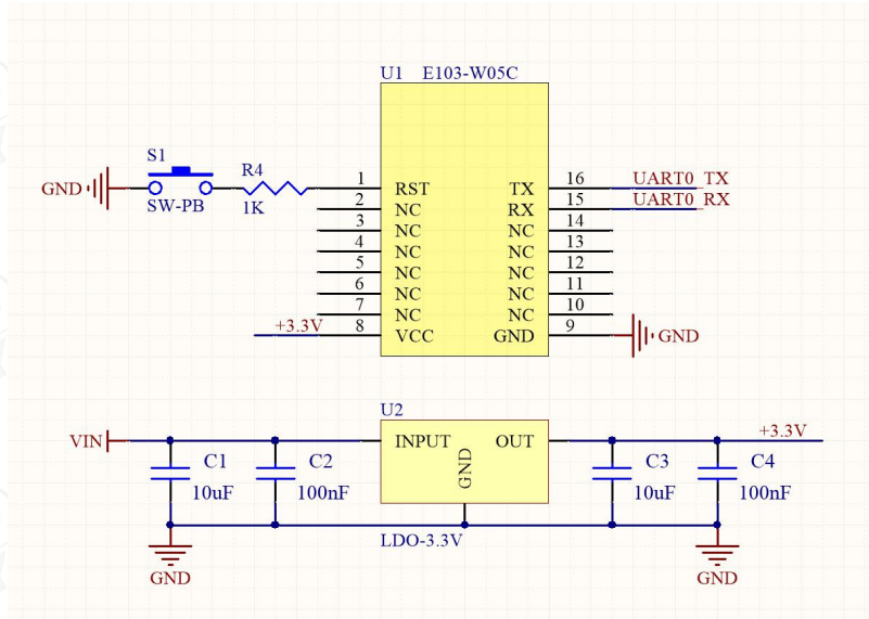
图 5-1 电路图
