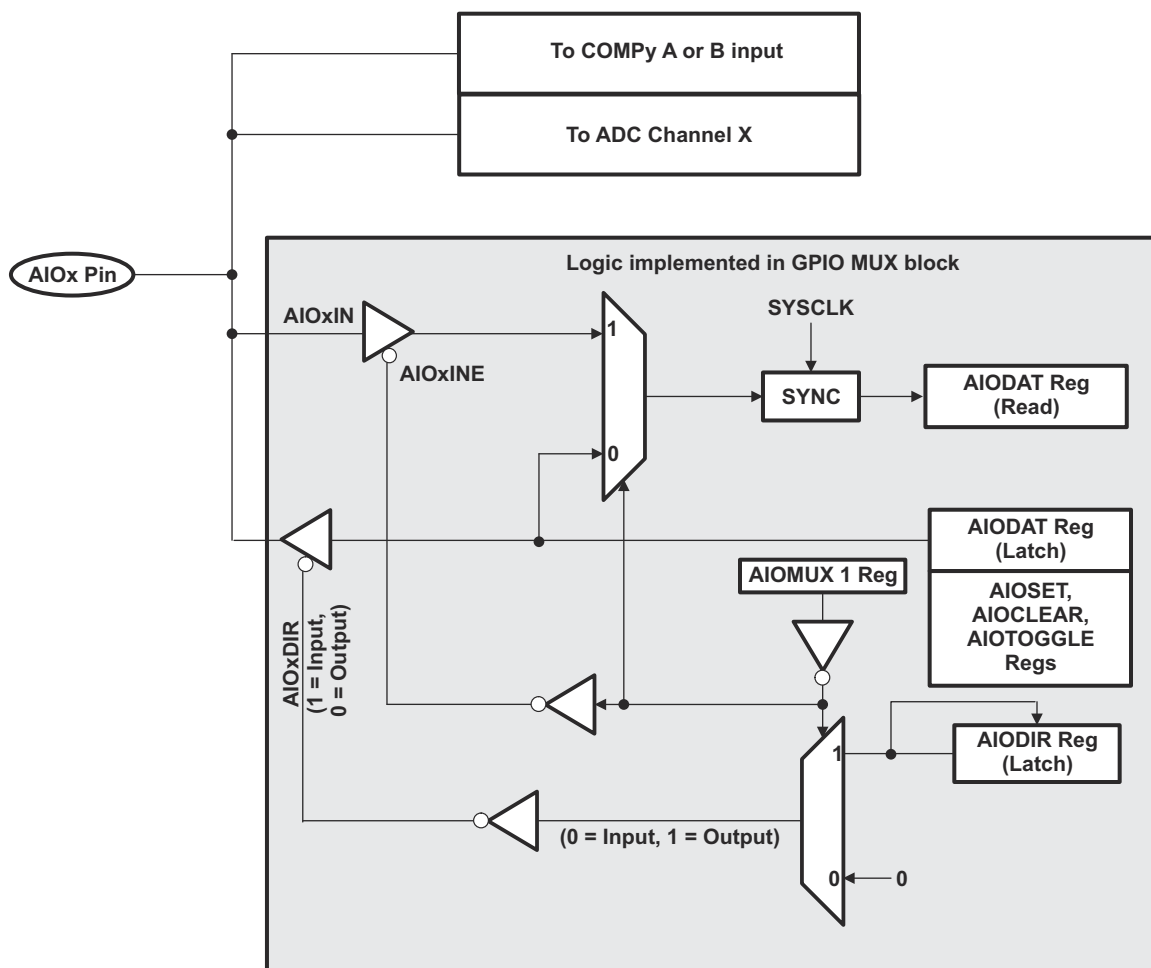
图 8-25. AIOx 引脚多路复用
