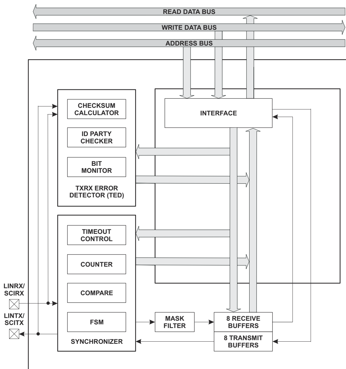
图 8-34. LIN 方框图
