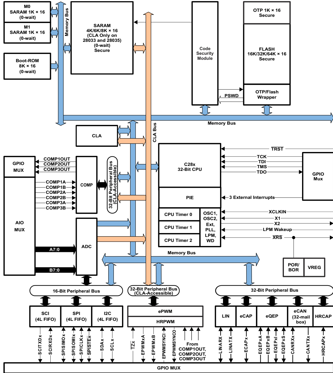
图 3-1. 功能方框图
