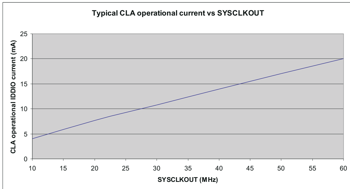
图 7-3. 典型 CLA 运行电流与 SYSCLKOUT 间的关系
