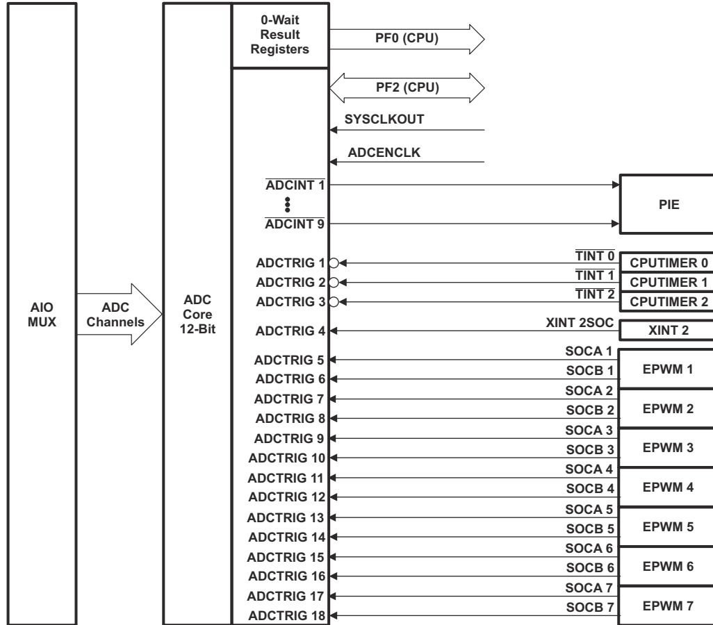
图 8-17. ADC 连接
