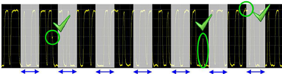
그림 10: InfiniiVision 3000T X-시리즈는 초당 100만 개의 파형을 지원합니다. 데드 타임이 짧기 때문에 간헐적 이벤트를 캡처할 수 있는 확률이 높습니다.
