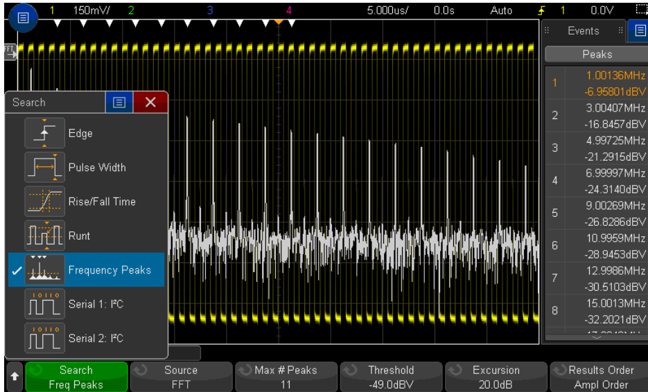
그림 14: 3000T X-시리즈는 FFT 분석을 위해 클럭 신호를 캡처하도록 설정되었습니다. 검색 및 탐색 기능을 이용하여 처음에 발생한 11개의 주파수 피크를 찾아서 탐색 삼각형으로 표시하고 신속하게 탐색할 수 있습니다. 그런 다음 주파수나 진폭의 순서대로 이를 정렬할 수 있습니다.
