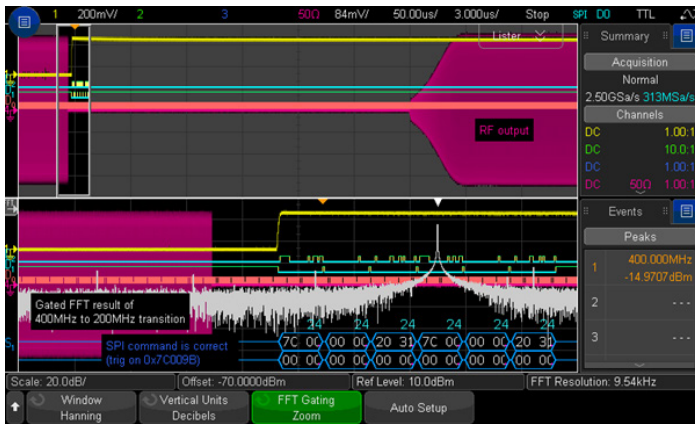
그림 21a: SPI 명령에서 트리거링된 RF 신호는 주파수 피크 검색 결과에 대한 lister 디스플레이에 표시되어 있듯이 여전히 400 MHz에 있습니다.
