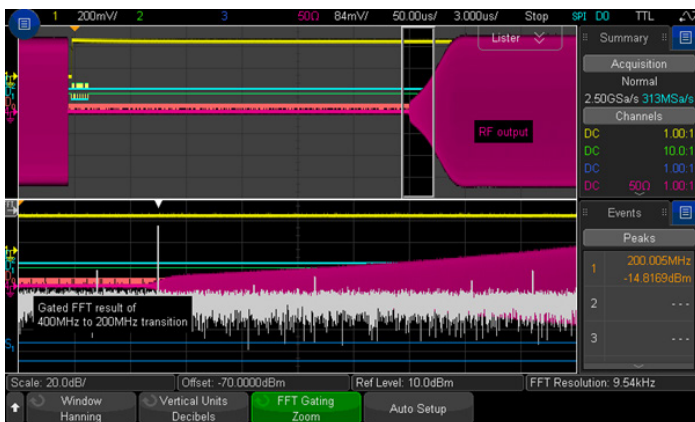
그림 21c: 200 MHz에서 RF 신호를 관찰하기 시작합니다. RF 아날로그 파형에서도 이를 검증할 수 있습니다.
