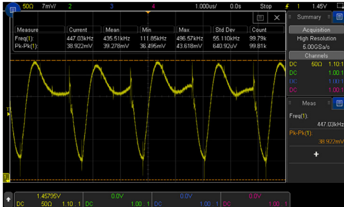
그림 30: 3000T X-시리즈와 N7020A는 전력 레일 리플 뿐만 아니라 고주파수 transient도 수집합니다.
