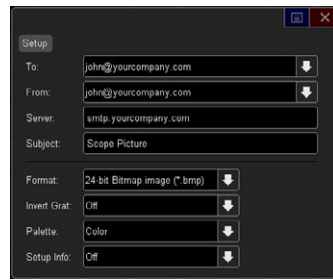
그림 6: LAN/VGA 모듈 옵션을 통해 측정 결과와 셋업, 데이터, 스크린샷을 자신의 이메일로 전송할 수 있습니다.
