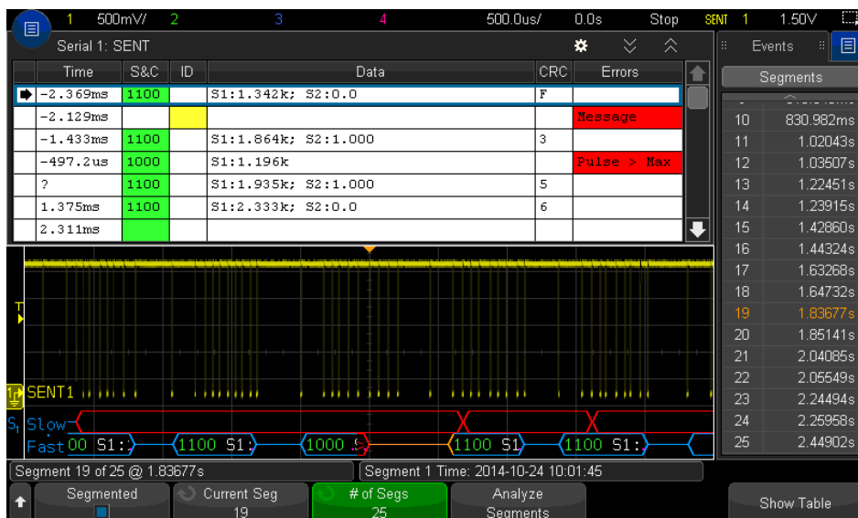
그림 20: 세그먼트화된 메모리가 시리얼 디코더와 함께 사용되기 때문에 시리얼 버스에 대한 정보를 최대한 얻을 수 있습니다.
