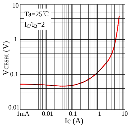
Fig5 VCESat-IC
