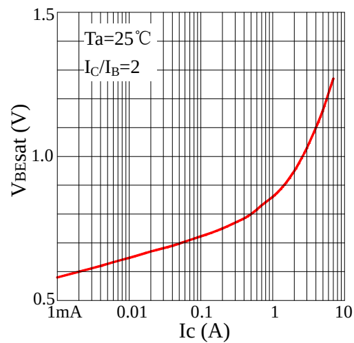
Fig6 VBEsat-IC
