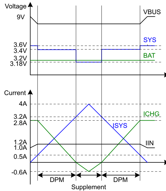
图 9. DPM Response
