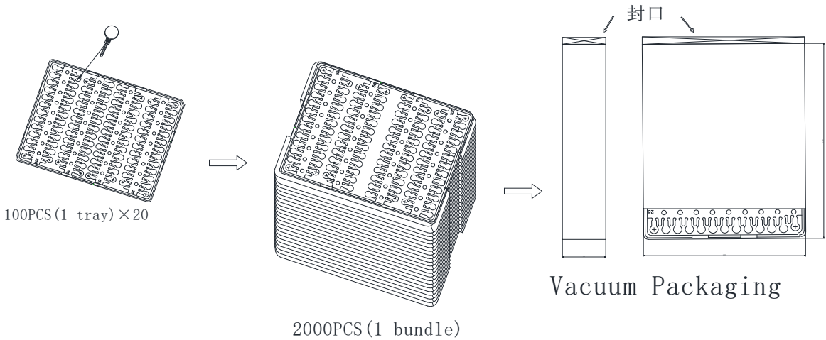
线性系列马达包装 Pack drawing of coin type
