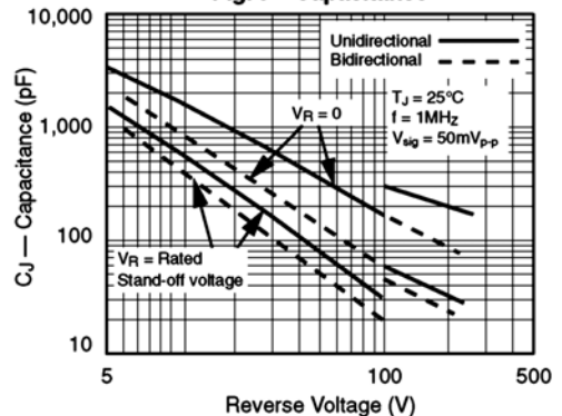
Fig. 6 – Capacitance
