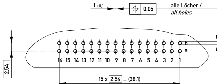
Leiterplatten- Lochbild / PCB drillhole pattern
