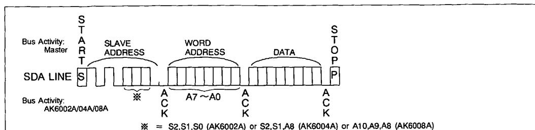
BYTE WRITE
