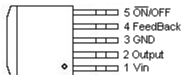
TO263-5L
