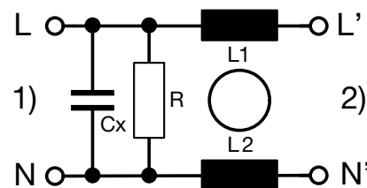
1) Line 2) Load
