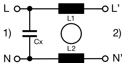
1) Line 2) Load
