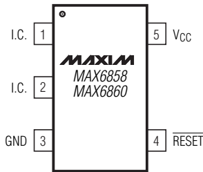
SOT23
