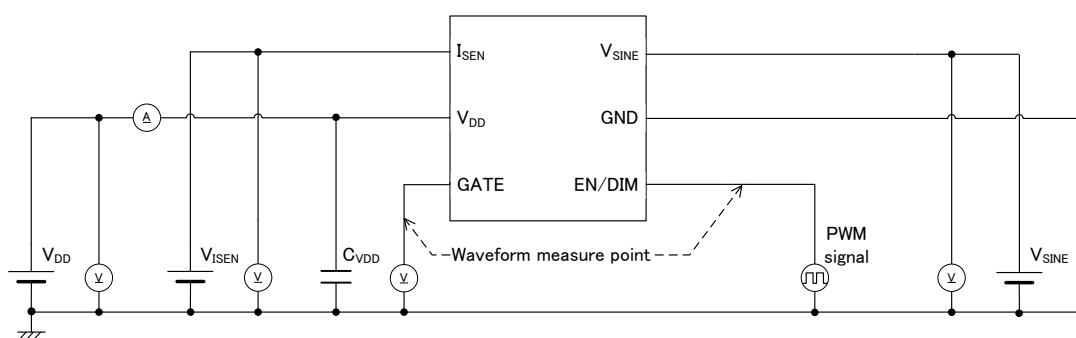
2) CIRCUIT②
