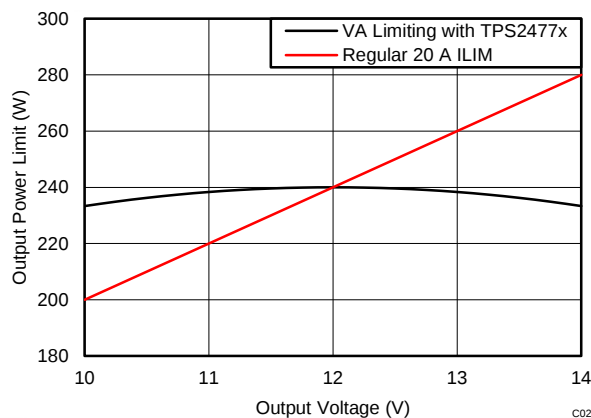
将输出功率限制在 240VA， 20A I LLIM 与 TPS2477x 实现的对比
