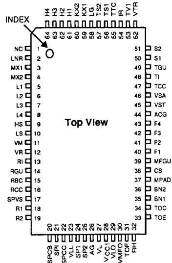
FPT-64P-M01
