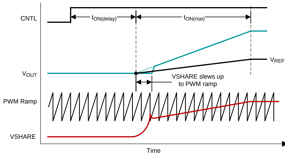
图 31. Soft-Start Timing
