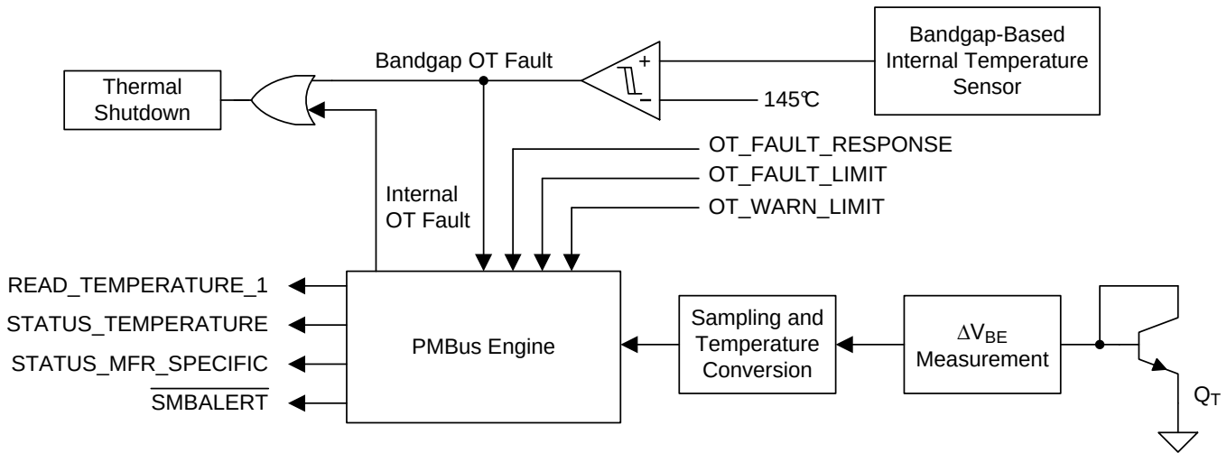
图 33. Overtemperature Protection
