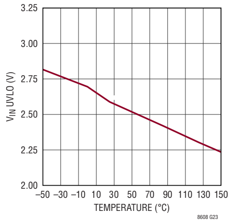
V_{\text{IN}} UVLO
