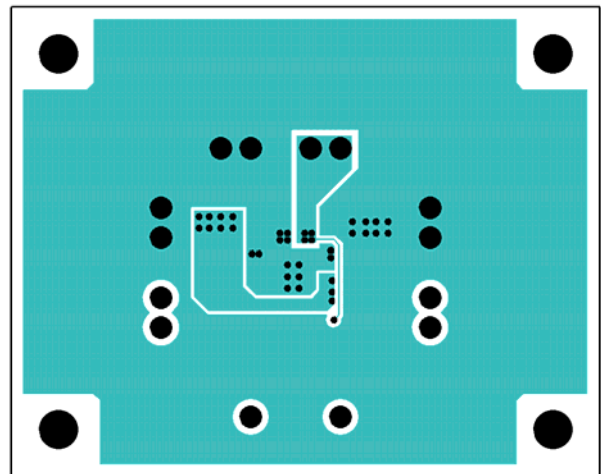
Bottom Side
