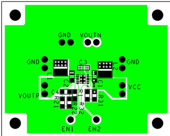
Top Side
