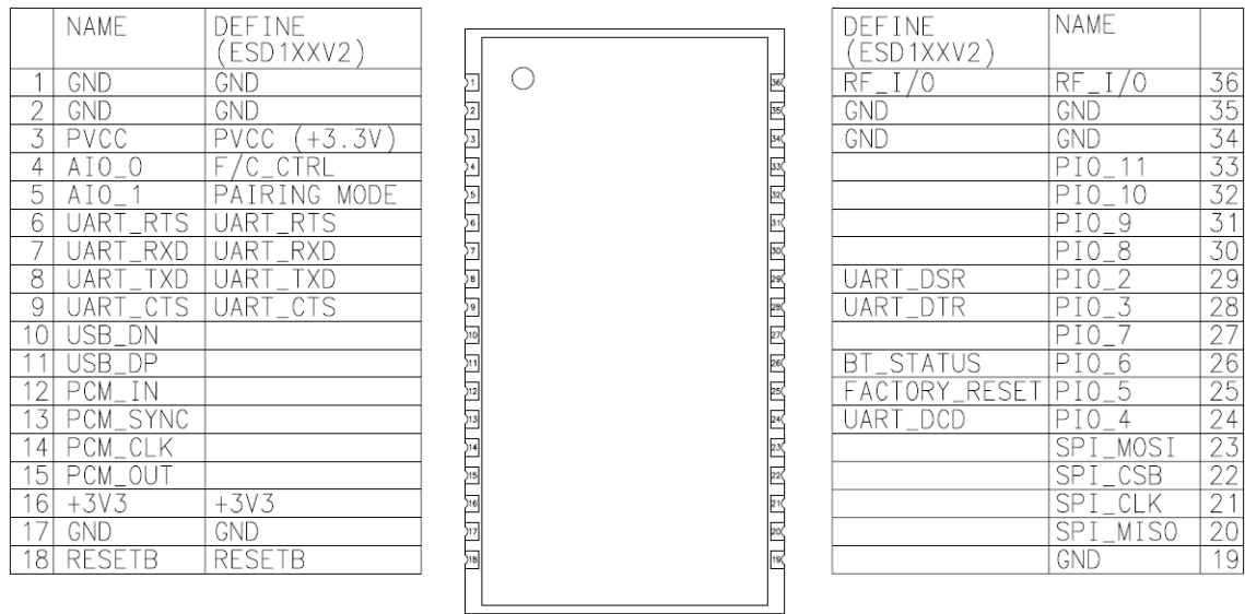
그림 1-2 핀 배치도
