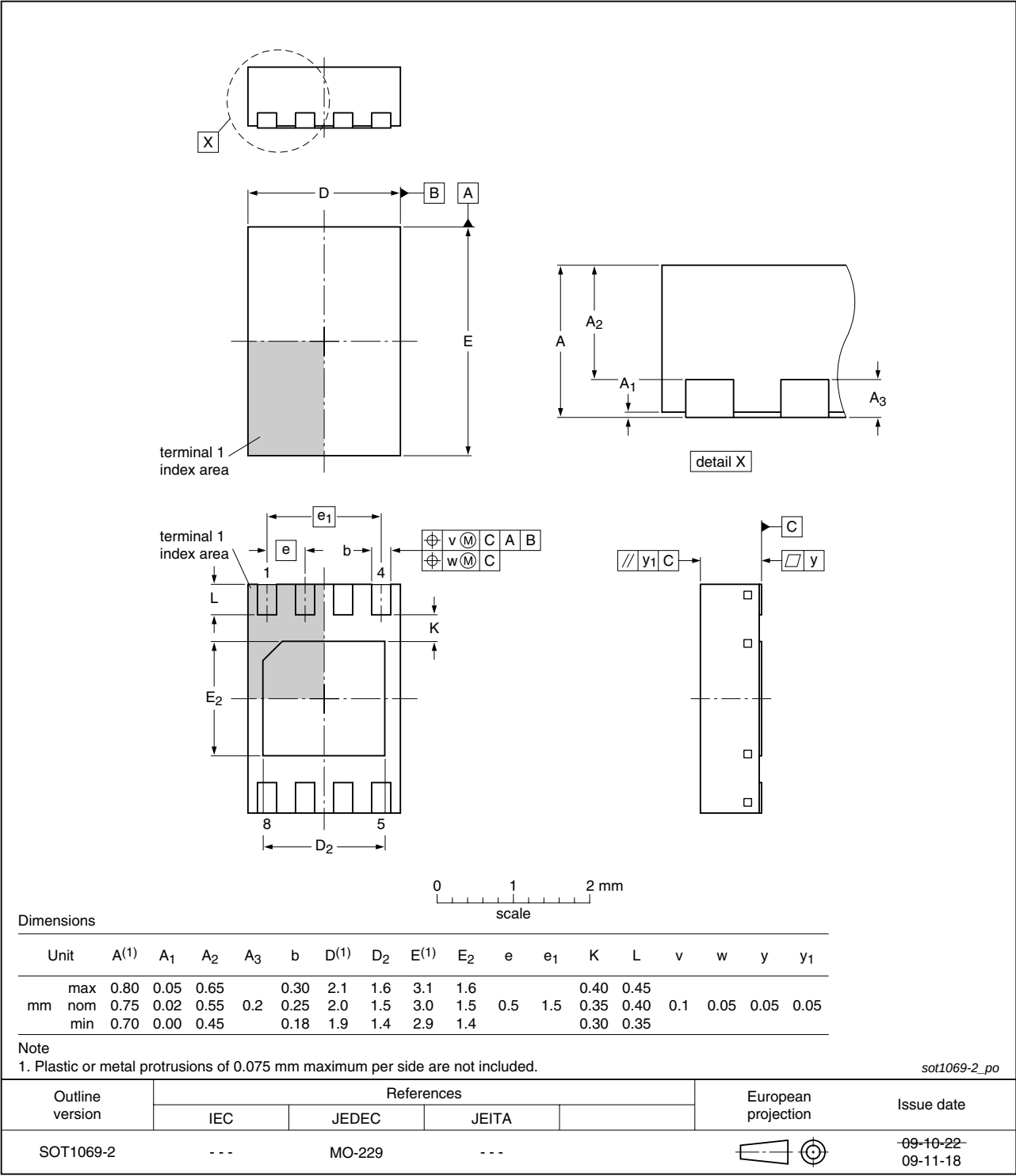
Fig 45. Package outline SOT1069-2 (HWSON8)
