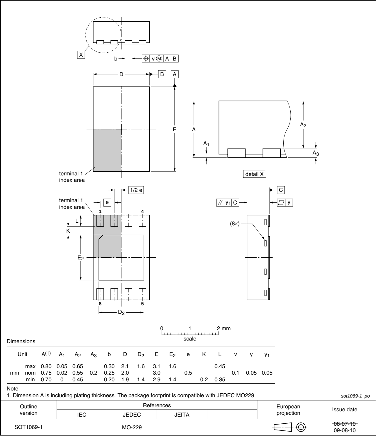
Fig 44. Package outline SOT1069-1 (HWSON8)
