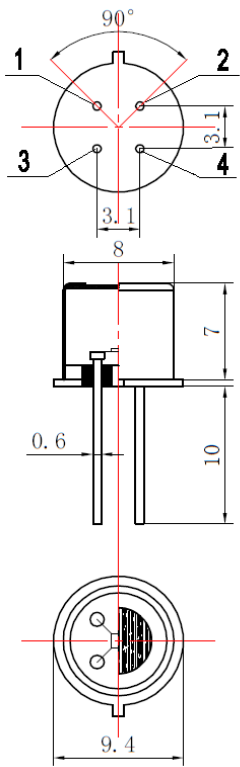
图 1: MP-2 外形结构图
