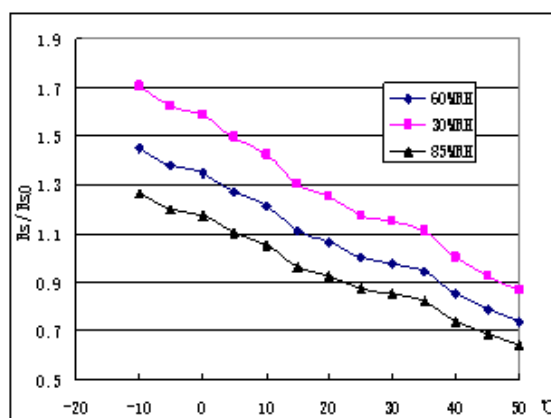
图 4 传感器典型的温度、湿度特性曲线
