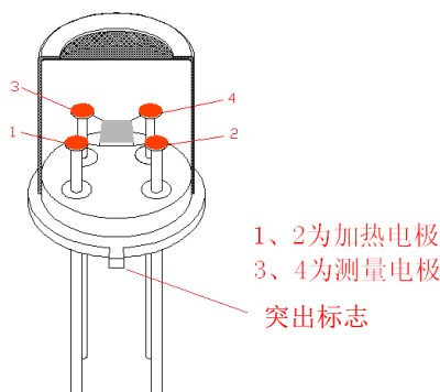
图 7： 管脚示意图
