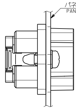
パネル後面取り付け REAR MOUNT TYPE
