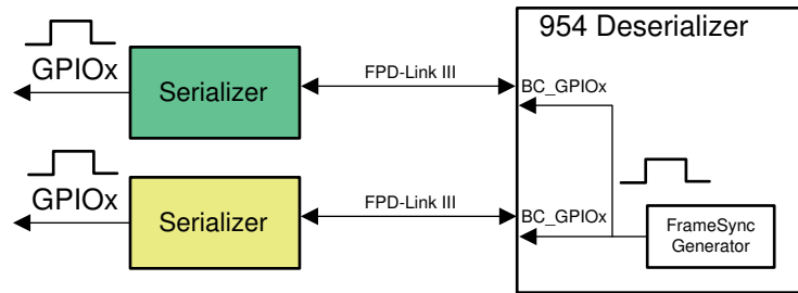
图 7-19. Internal FrameSync
