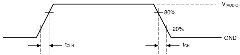
图 6-1. LVCMOS Transition Times
