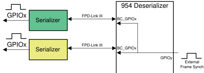
图 7-17. External FrameSync
