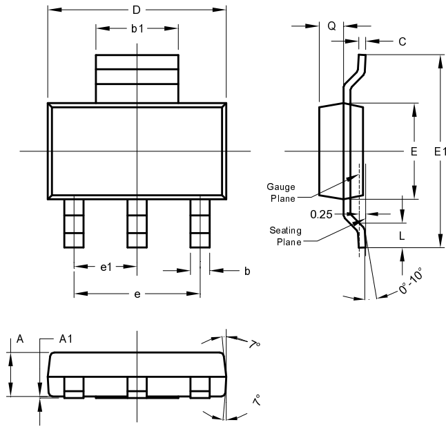
SOT223
