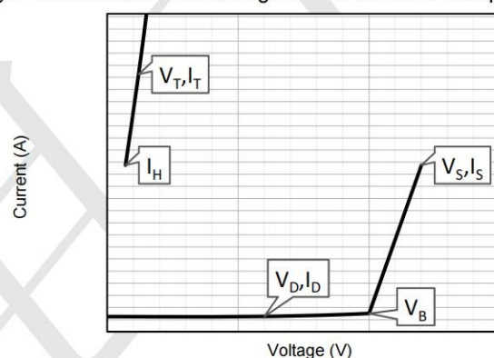
Fig.4 - VI Curve
