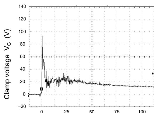
Fig. 10.1 +8 kV
