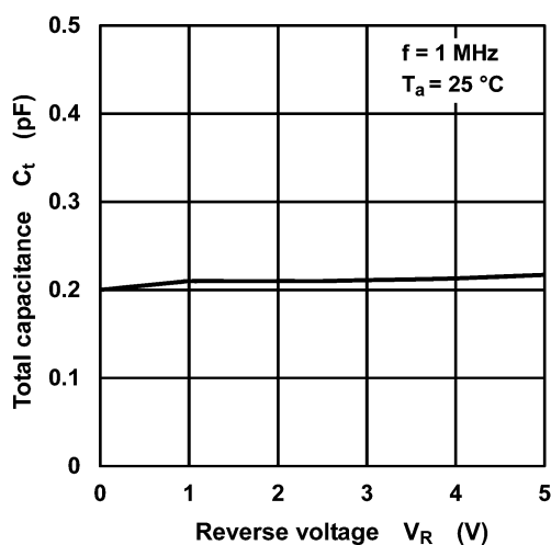
Fig. 7.3 C_t - V_R
