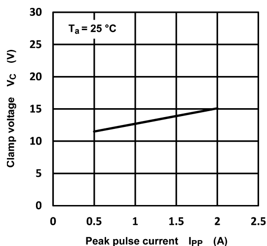
Fig. 8.1 V_C - I_{PP}
