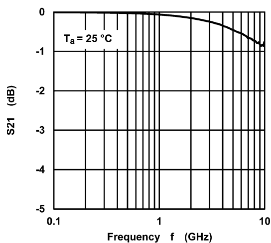
Fig. 9.1 S_{21} - f
