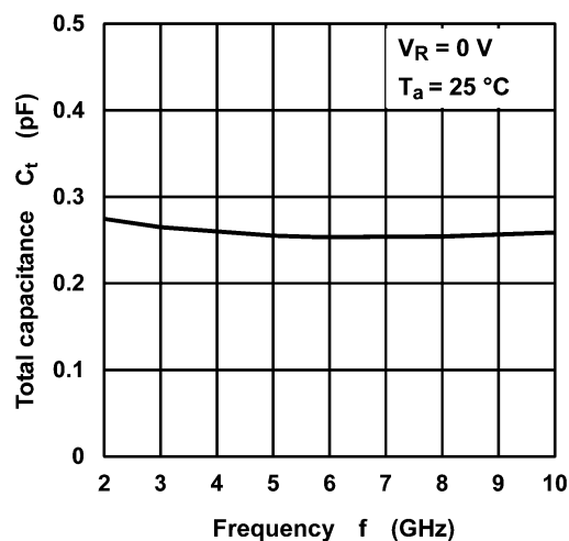
Fig. 7.4 C_t - f
