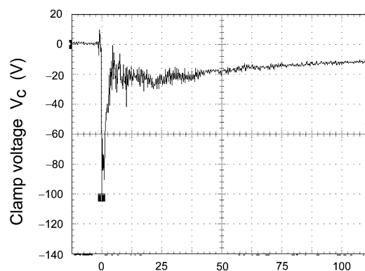
Fig. 10.2 -8 kV
