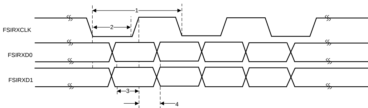
图 5-88. FSIRX Timings
