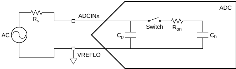
图 5-34. Input Model
