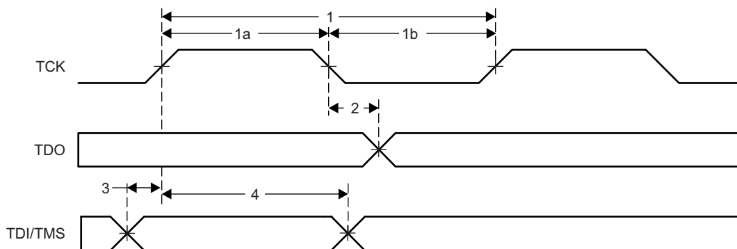
图 5-19. JTAG Timing
