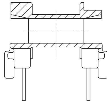
SEC. A-A
