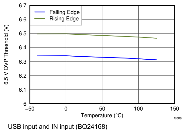
图 7-6. 6.5-V OVP Threshold vs Temperature
