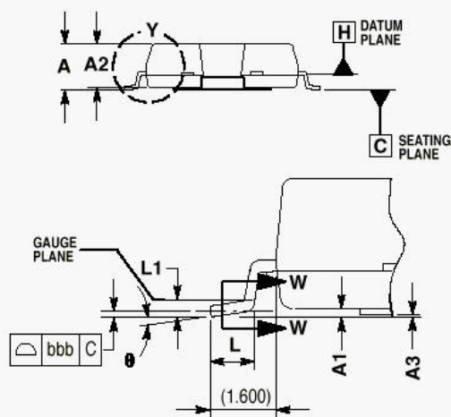
DETAIL Y
