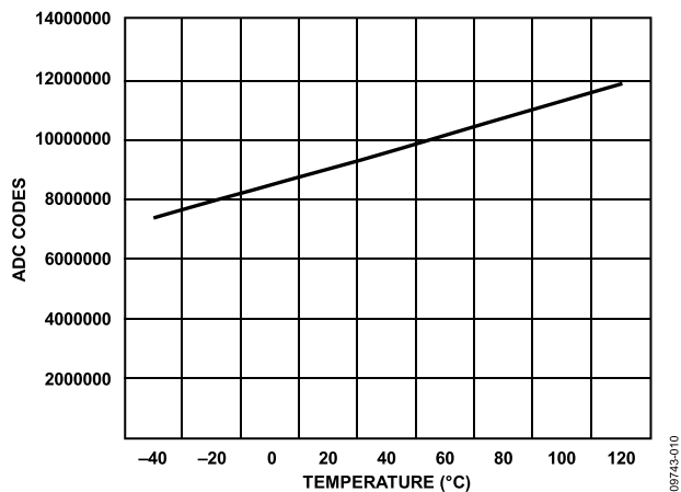
图11. ADC代码(十进制数值)与芯片温度的关系, 测量仪针对温度传感器
