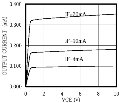
I_o vs V_{CE}
