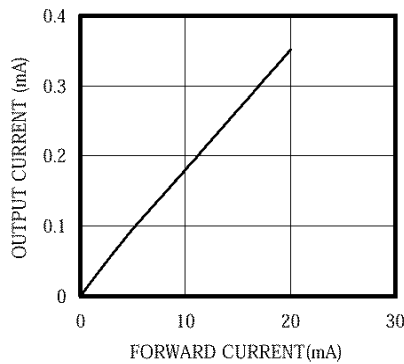
I_F vs I_o V_{CE}=10V
