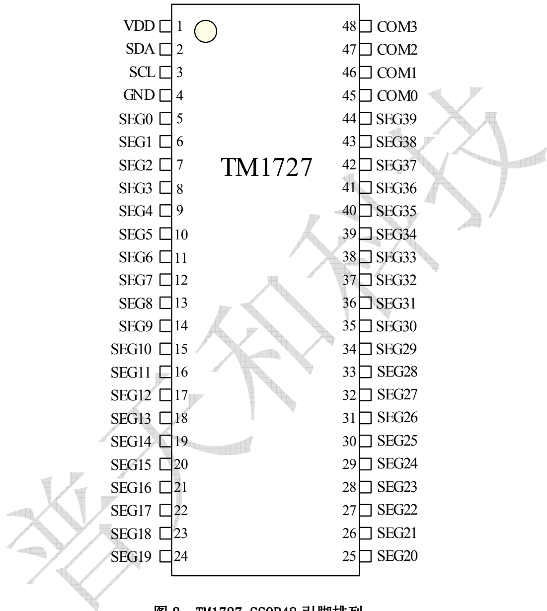
图 2：TM1727-SSOP48 引脚排列
