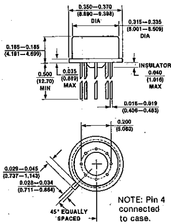
TO-99 (TV)
