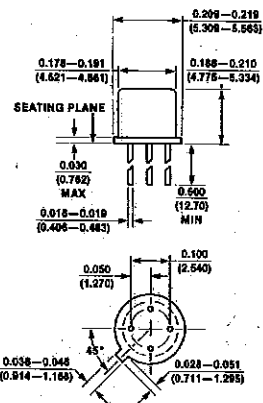
TO-72 (US)
