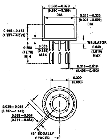
TO-99 (TV)
