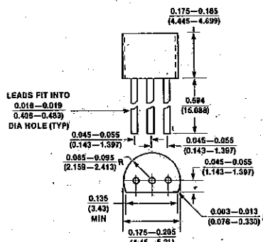
TO-92 (ZR)
