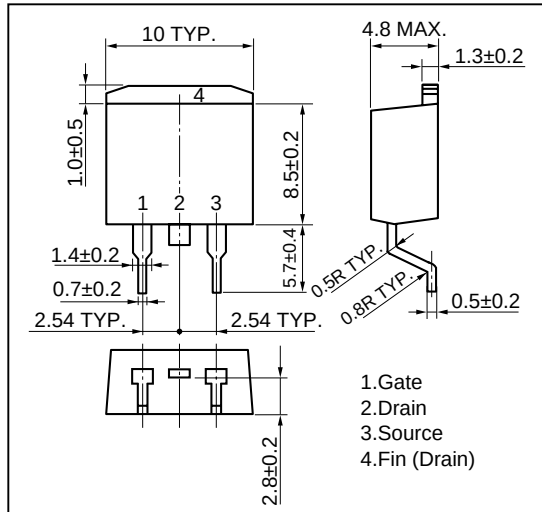
3) TO-263 (MP-25ZJ)
