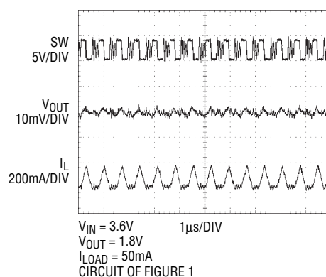
PWM Mode
