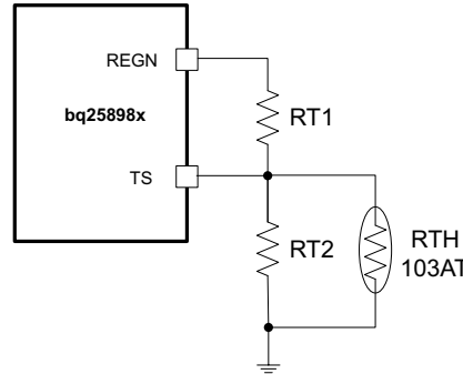
图 16. TS Resistor Network
