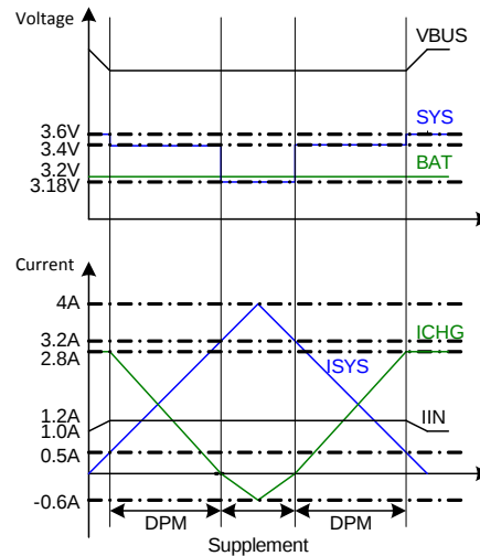
图 13. DPM Response
