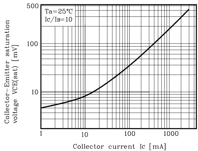
Fig. 1 V_{CE(sat)} - I_C
