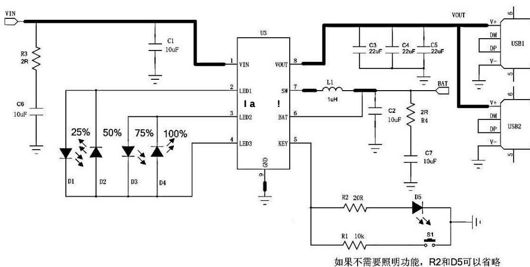
图 1 简化应用原理图(4 LED 指示电量)
