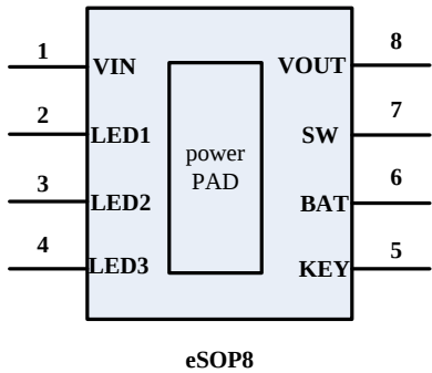
图 2 （ - ）!引脚图
