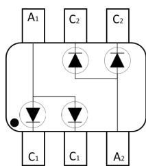
BAS40ADW
